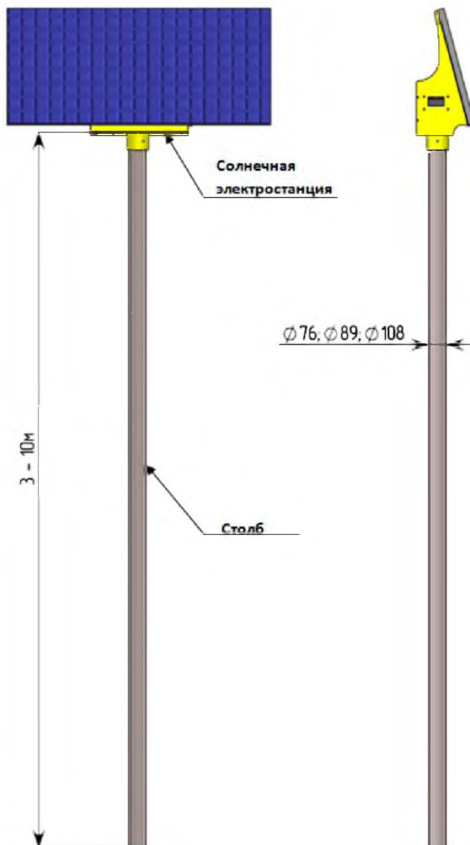
Рисунок 4. Установка солнечной электростанции «GM».
